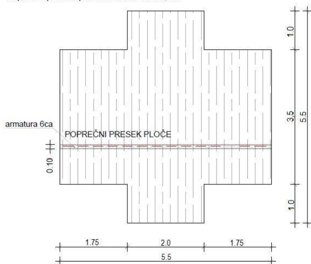
Poprečni presek ploče bazena 5x3x1,2m
