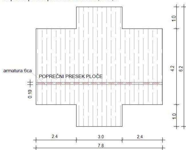
Poprečni presek ploče bazena 7.3x3.75x1,2
