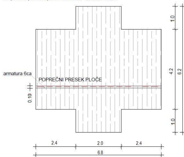
Poprečni presek ploče bazena 6,1x3,75x1,2
